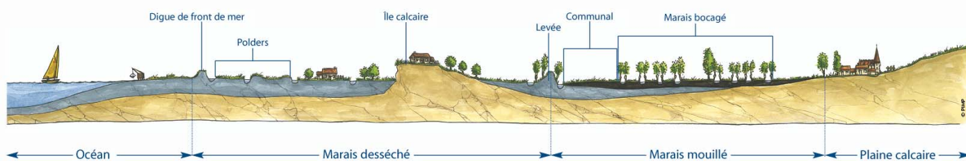
UP49-20-14bis Coupe de principe d'organisation des marais (Source PNR Marais poitevin © PIMP)
