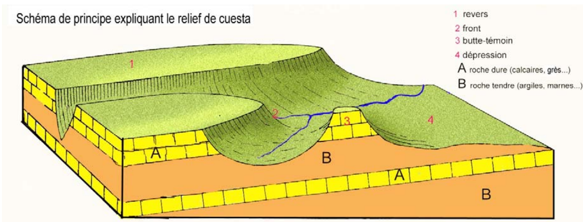
UP10-20-03 Schéma de principe expliquant le relief de cuesta
