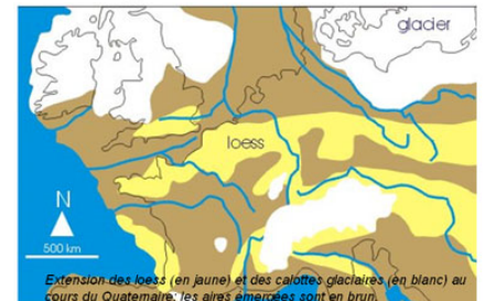
UP34-20-03 Schéma de principe de formation géologique au cénozoïque (source Atlas des paysages de Loire-Atlantique 2010)
