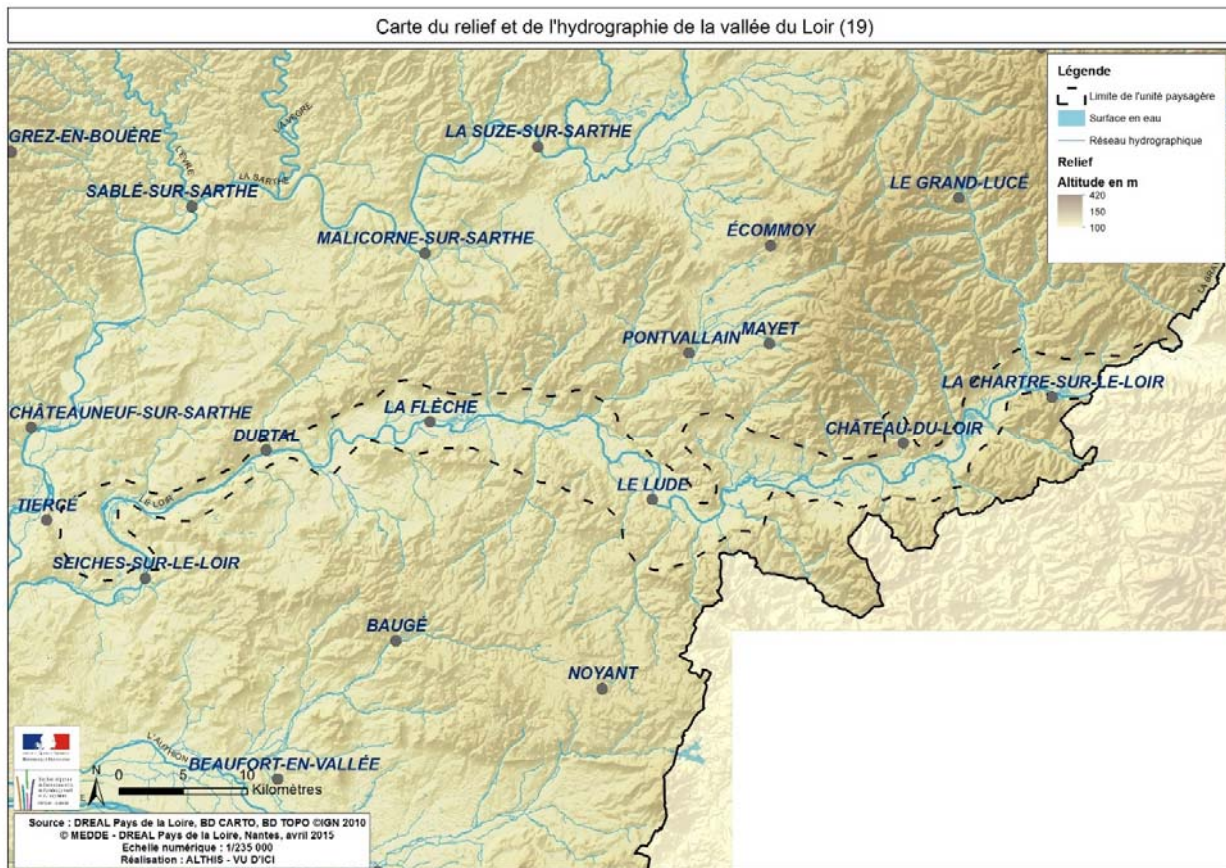
UP19-20-C2 Carte du relief et du réseau hydrographique de la vallée du Loir
