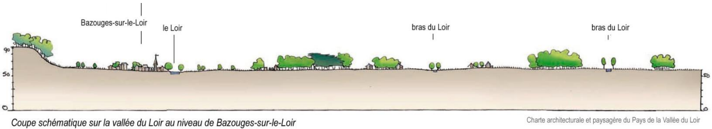
Coupe schématique sur la vallée du Loir au niveau de Bazouges-sur-le-Loir
