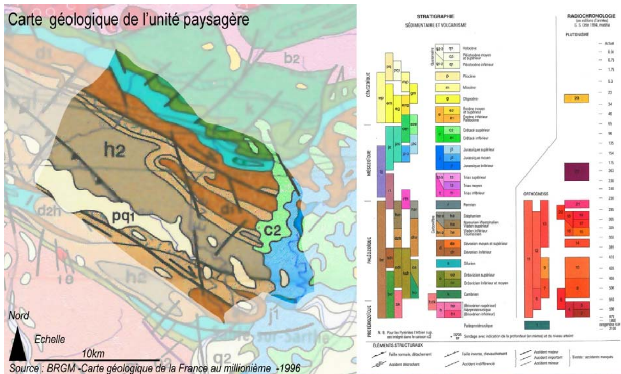
UP07-20-02 Extrait de carte géologique de l'unité paysagère du Bas-Maine (source : BRGM)
