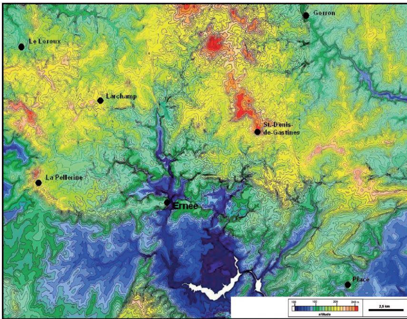
UP01-20-C3 Fig. 1 – Modelé du relief à partir du MNT de la feuille d'Ernée (source BRGM)
