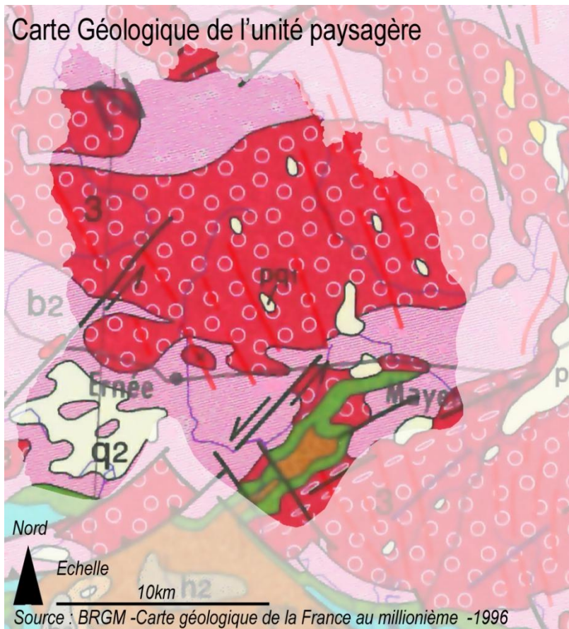
UP01-20-C1 Carte géologique de l'unité paysagère des marches entre Maine et Bretagne
